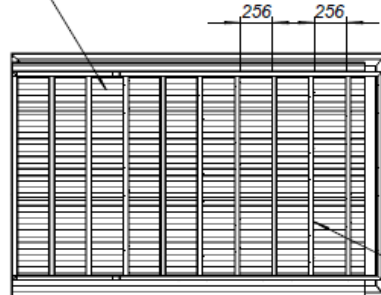
SECCIÓN F-F
